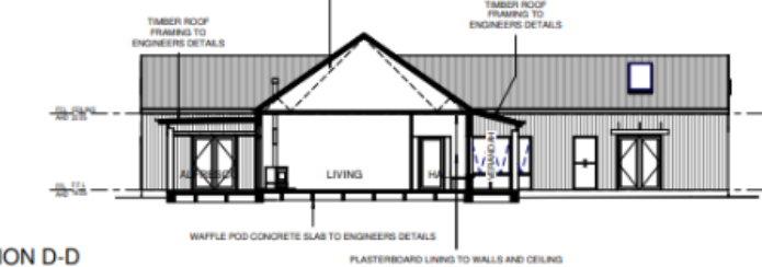
SECTION D-D
